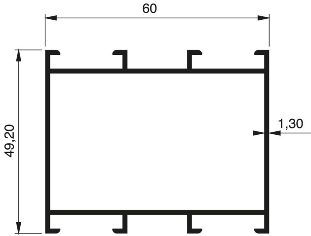
915 - 0.892 Kg/m
