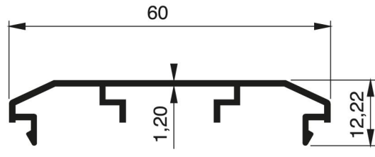
904 - 0.344 Kg/m
