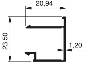
903 - 0.229 Kg/m
