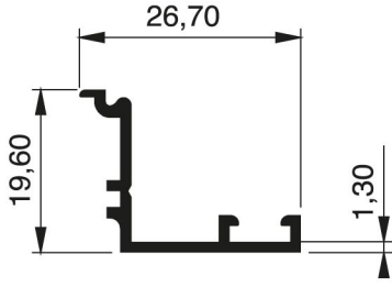
900 - 0.206 Kg/m
