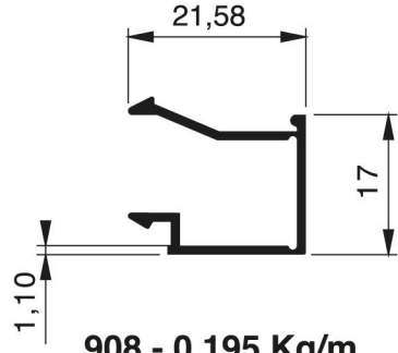
908 - 0.195 Kg/m
