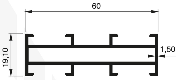
907 - 0.761 Kg/m
