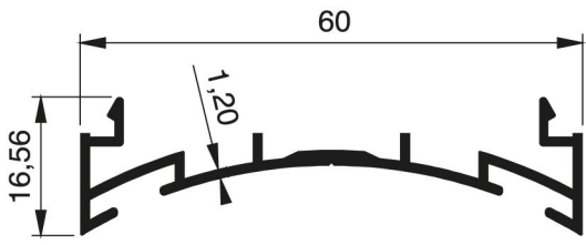
909 - 0.430 Kg/m
