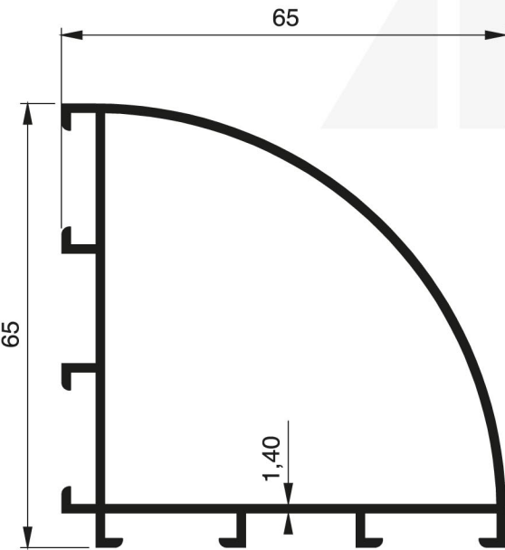
906 - 1.017 Kg/m
