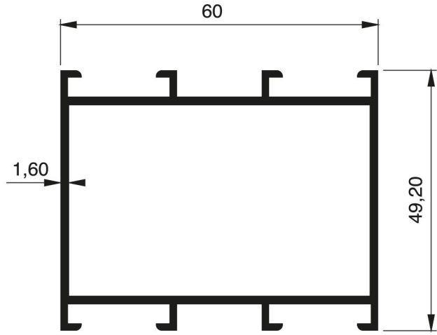
901 - 1.056 Kg/m
