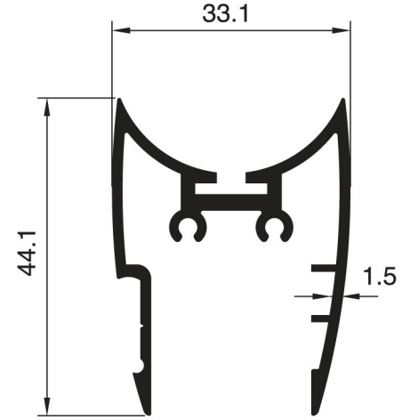
2159 - 0.710 Kg/m
