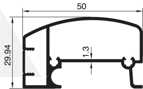
2381 - 0.691 Kg/m
