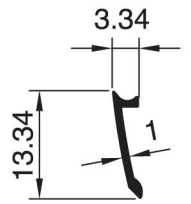
2368 - 0.044 Kg/m
