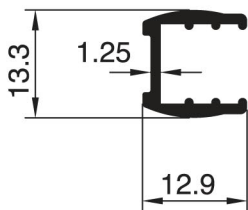
2462 - 0.146 Kg/m
