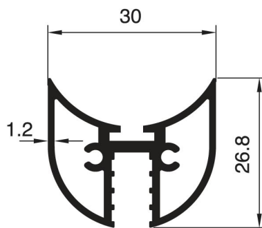
2162 - 0.545 Kg/m
