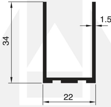
2209 - 0.374 Kg/m
