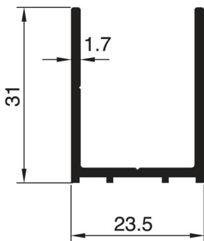
2482 - 0.384 Kg/m
