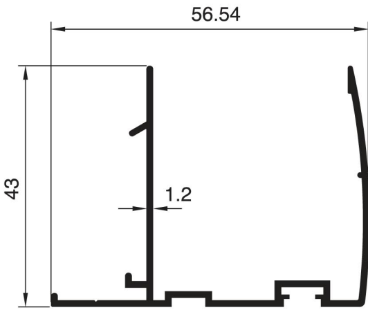
1026 - 0.530 Kg/m
