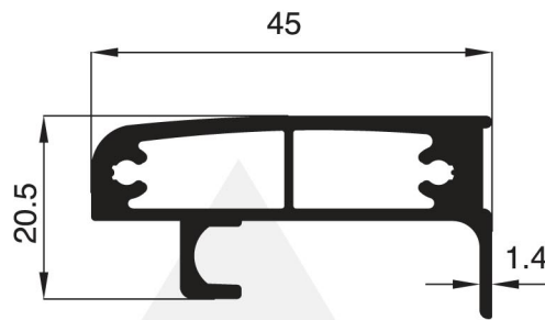
2269 - 0.739 Kg/m
