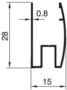
2408 - 0.192 Kg/m
