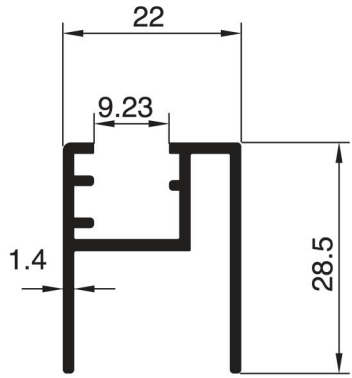
2506 - 0.372 Kg/m
