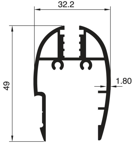
2158 - 0.775 Kg/m
