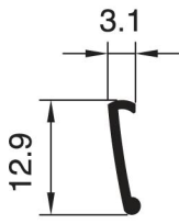
2218 - 0.045 Kg/m
