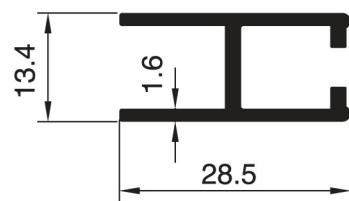
1901 - 0.330 Kg/m
