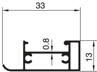
2407 - 0.246 Kg/m
