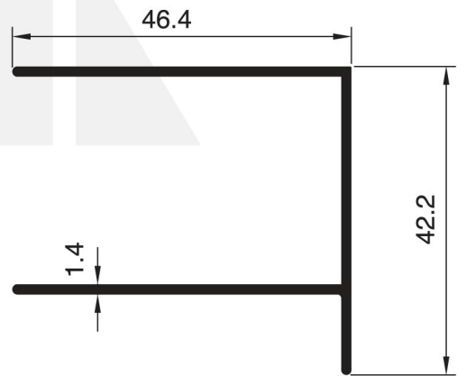
1263 - 0.500 Kg/m
