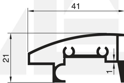
2378 - 0.448 Kg/m
