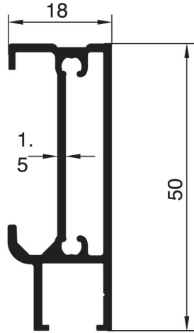
2504 - 0.600 Kg/m
