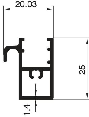
2503 - 0.356 Kg/m
