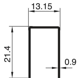
2389 - 0.131 Kg/m
