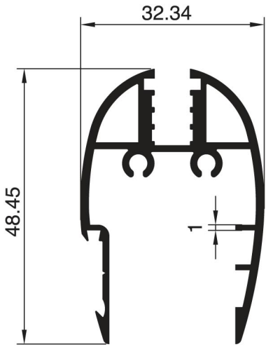
2367 - 0.765 Kg/m
