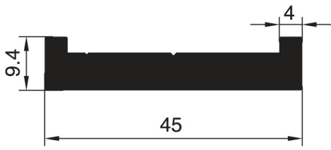
2380 - 0.864 Kg/m
