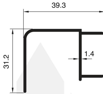
1283 - 0.385 Kg/m
