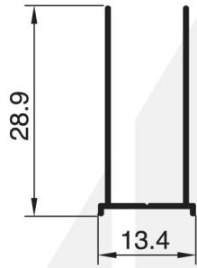
2409 - 0.150 Kg/m
