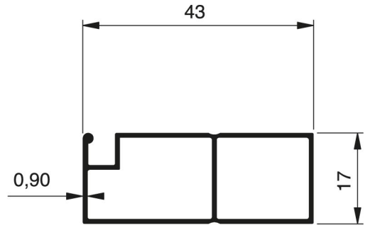
2032 - 0.350 Kg/m
