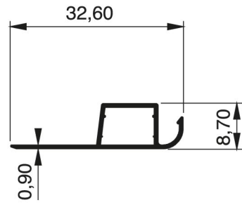
752 - 0.150 Kg/m
