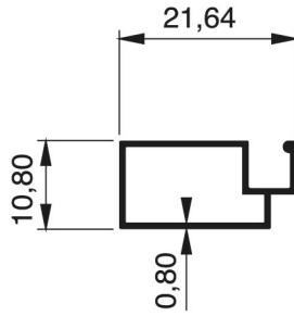
751 - 0.142 Kg/m
