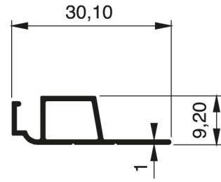
753 - 0.168 Kg/m
