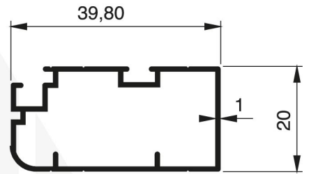
756 - 0.369 Kg/m
