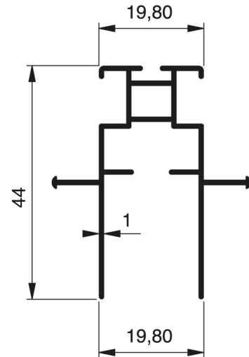
1959 - 0.458 Kg/m
