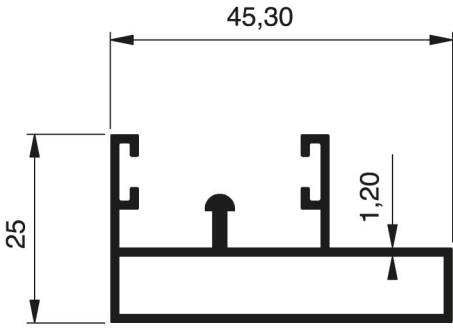
1824 - 0.545 Kg/m
