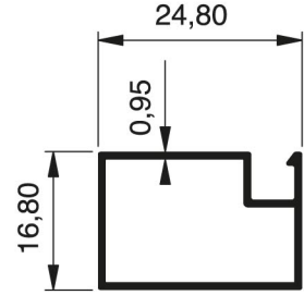
757 - 0.222 Kg/m
