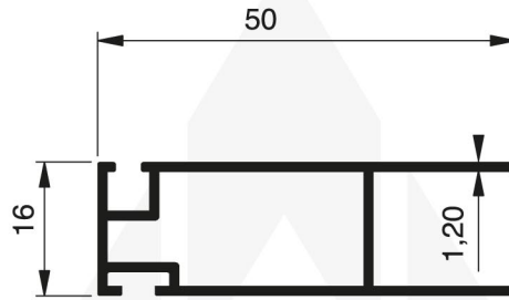
1825 - 0.458 Kg/m
