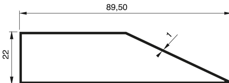
1002 - 0.550 Kg/m
