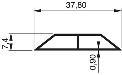
997 - 0.201 Kg/m
