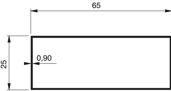
1000 - 0.430 Kg/m
