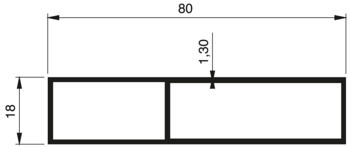
1148 - 0.714 Kg/m
