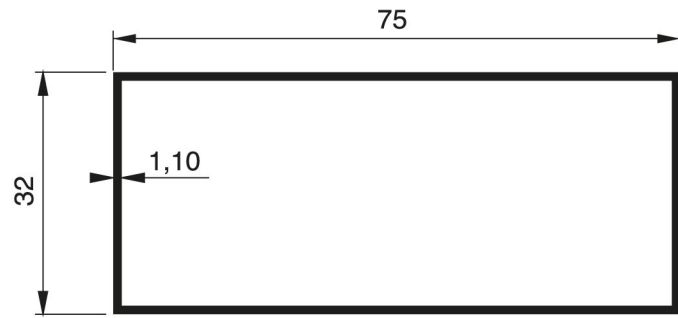
998 - 0.625 Kg/m
