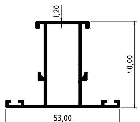
4049 - 0.602 Kg/m
