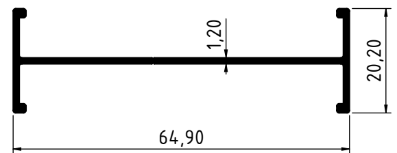
4181 - 0.361 Kg/m
