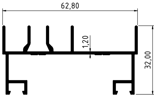
4045 - 0.648 Kg/m
