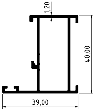
4047 - 0.524 Kg/m
