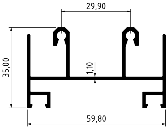
4042 - 0.729 Kg/m
