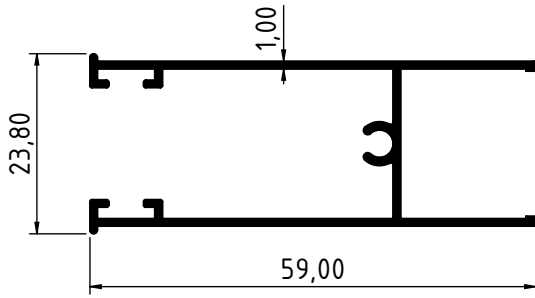
2353 - 0.450 Kg/m
