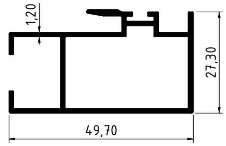
4044 - 0.599 Kg/m
