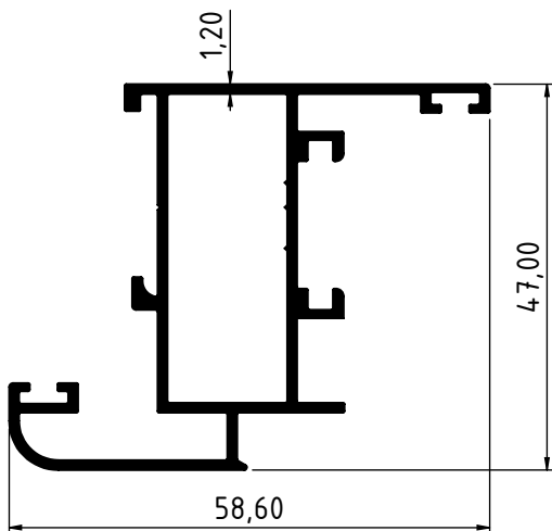
4047 - 0.524 Kg/m
