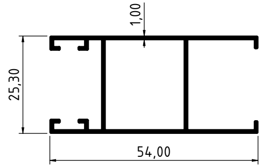
2355 - 0.480 Kg/m
