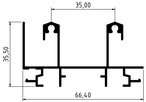
2354 - 0.738 Kg/m
