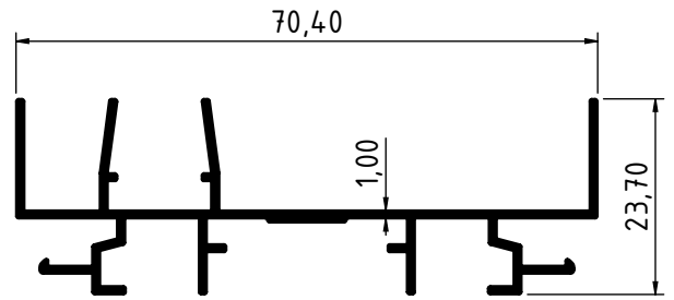
2356 - 0.537 Kg/m
