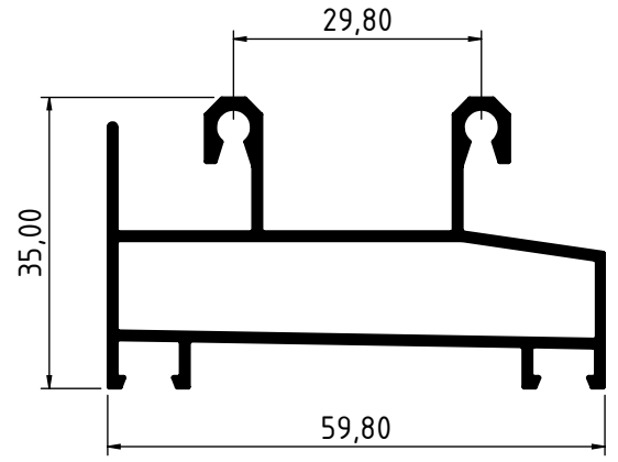
4039 - 0.786 Kg/m
