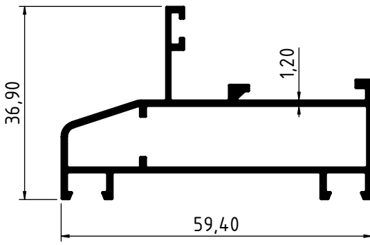
4043 - 0.640 Kg/m
