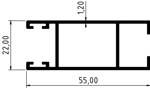
4040 - 0.572 Kg/m
