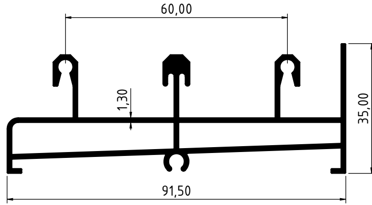
6895 - 1.258 Kg/m
