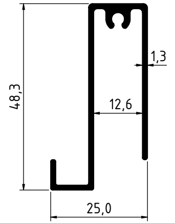
2744 - 0.469 Kg/m
