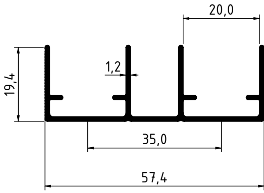
1060 - 0.466 Kg/m
