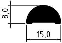
3272 - 0.247 Kg/m
