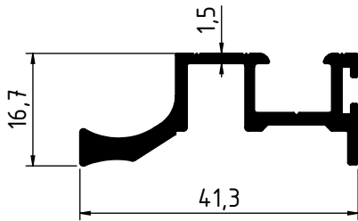
2747 - 0.445 Kg/m
