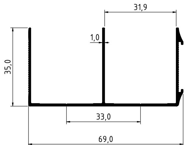
2581 - 0.500 Kg/m
