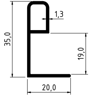
2268 - 0.286 Kg/m
