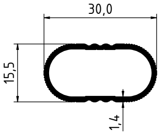
2901 - 0.244 Kg/m
