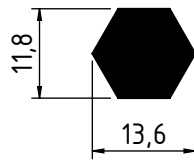
2305 - 0.328 Kg/m
