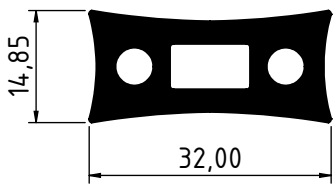
2171 - 0.805 Kg/m
