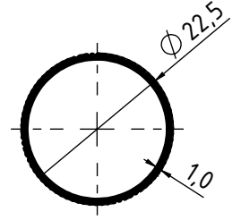
2416 - 0.165 Kg/m
