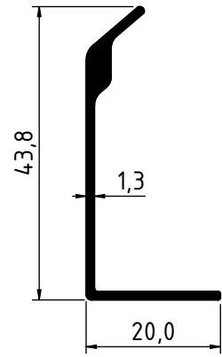
3072 - 0.266 Kg/m
