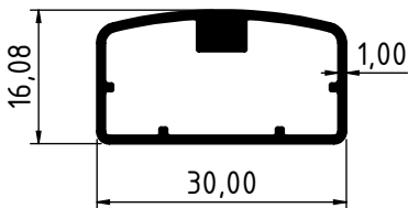
3482 - 0.301 Kg/m
