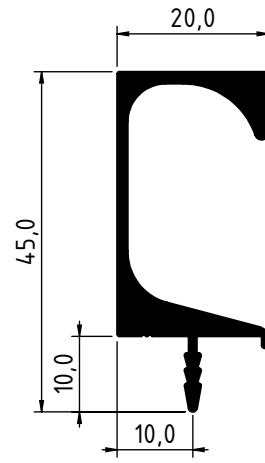
2708 - 0.540 Kg/m
