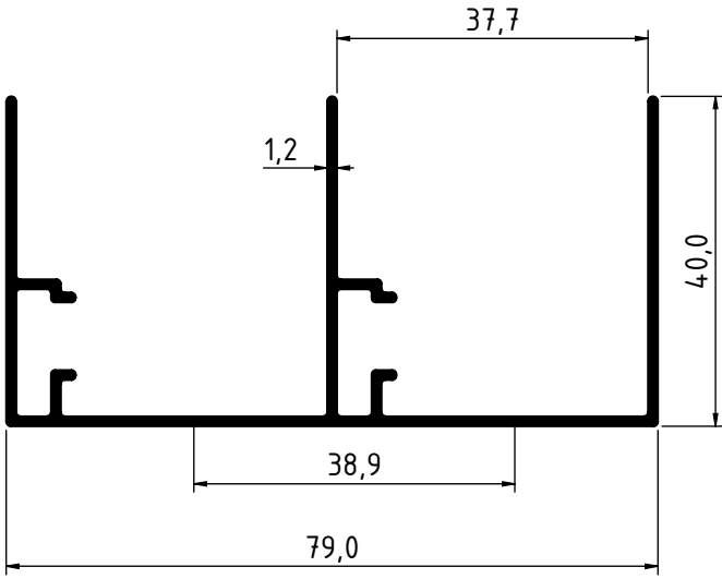
3973 - 0.746 Kg/m
