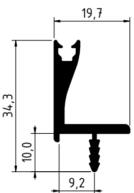
2719 - 0.385 Kg/m
