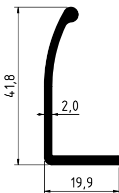
3837 - 0.363 Kg/m
