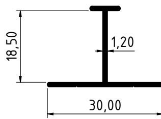
2973 - 0.181 Kg/m
