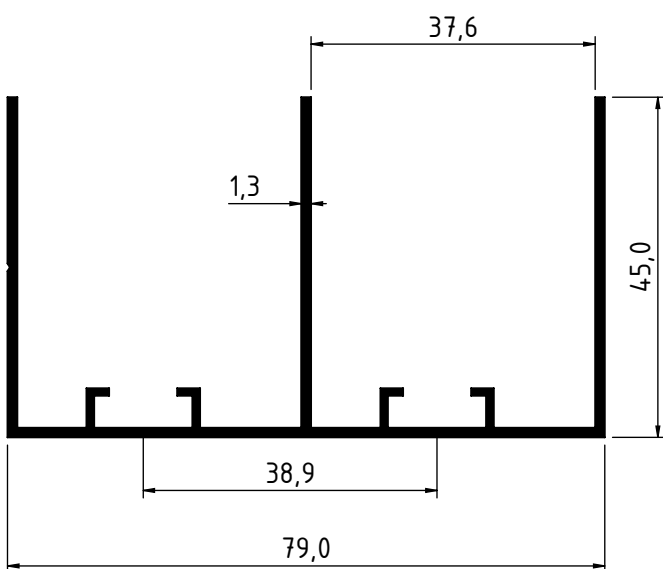
1217 - 0.818 Kg/m
