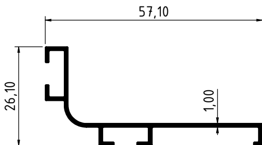
2717 - 0.304 Kg/m
