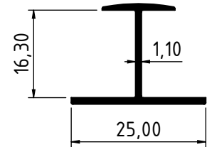
3011 - 0.169 Kg/m
