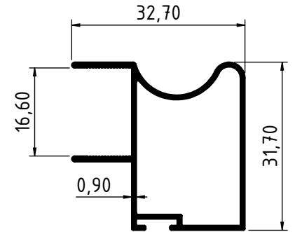
3237 - 0.401 Kg/m
