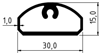
3910 - 0.320 Kg/m
