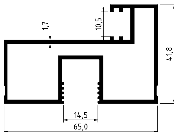
1968 - 1.030 Kg/m
