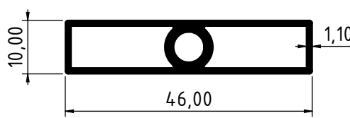
3733 - 0.418 Kg/m
