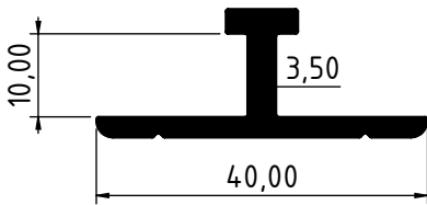
3519 - 0.431 Kg/m
