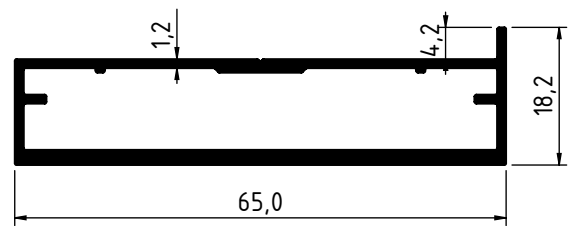
4018 - 0.690 Kg/m
