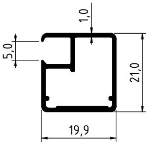
1888 - 0.259 Kg/m
