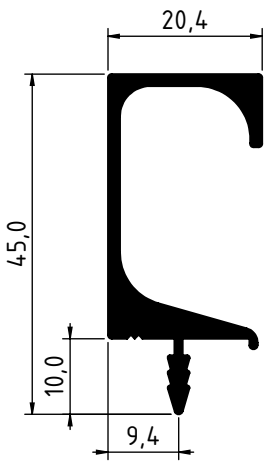
2612 - 0.550 Kg/m
