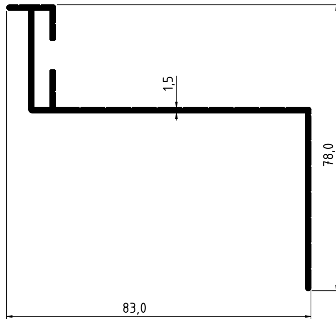
2767 - 0.740 Kg/m
