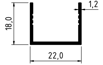
2553 - 0.176 Kg/m
