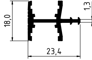
3293 - 0.250 Kg/m
