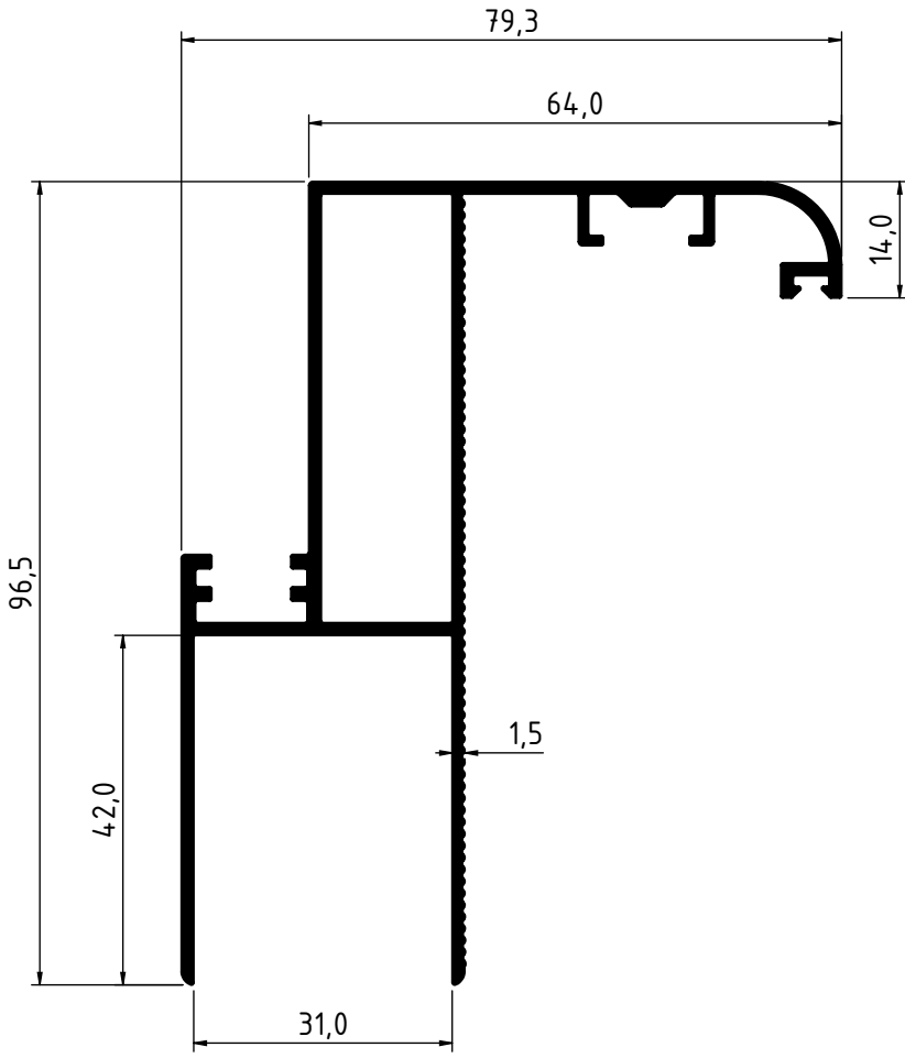
4443 - 1.345 Kg/m
