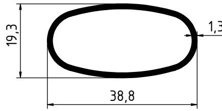
3058 - 0.328 Kg/m
