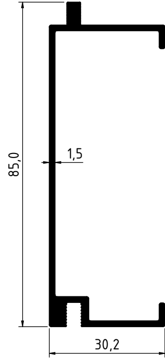
4444 - 0.732 Kg/m
