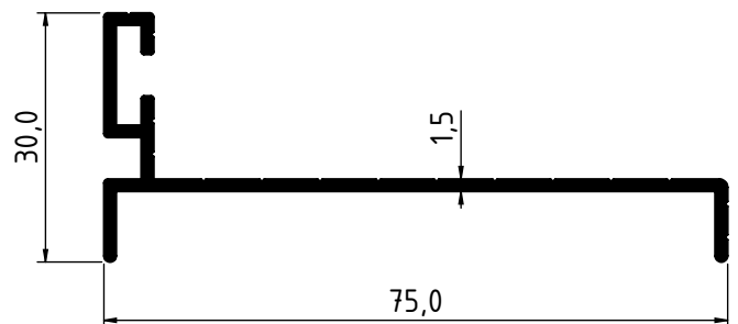
2769 - 0.518 Kg/m
