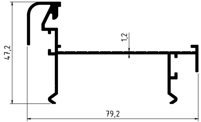
2983 - 0.718 Kg/m
