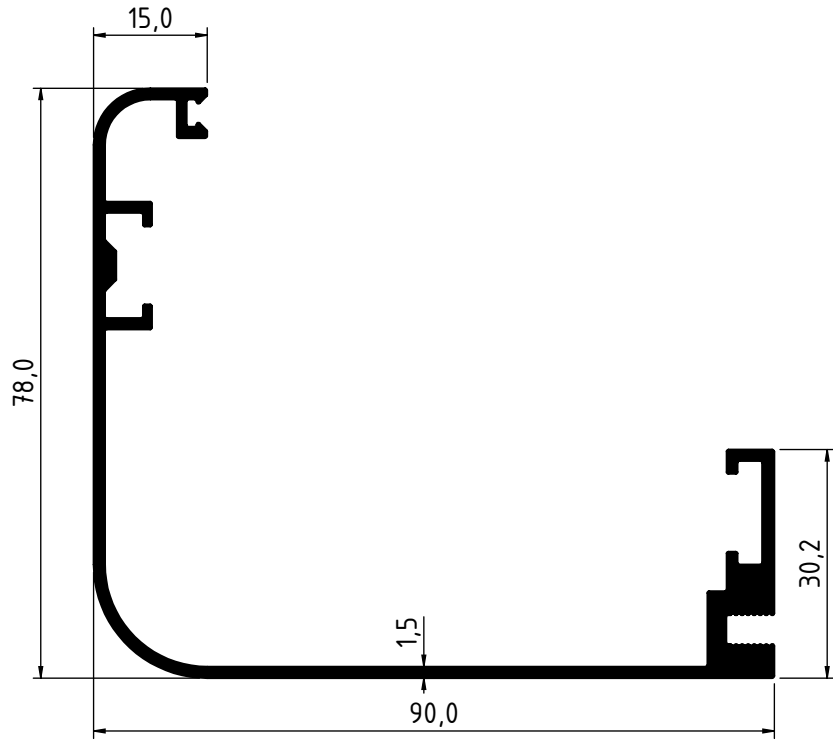
4446 - 1.138 Kg/m
