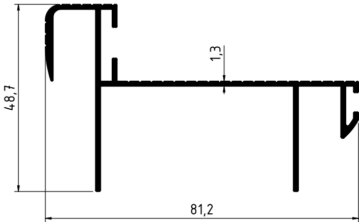
2467 - 0.762 Kg/m
