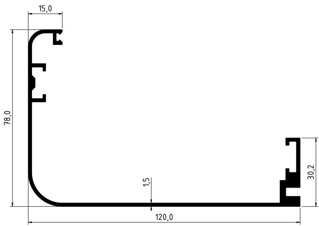
4445 - 1.260 Kg/m
