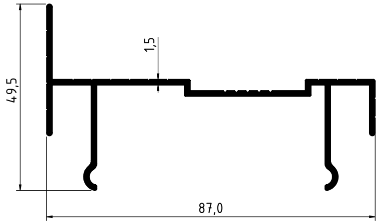
2768 - 0.805 Kg/m
