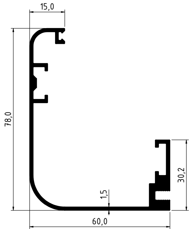
4447 - 1.016 Kg/m
