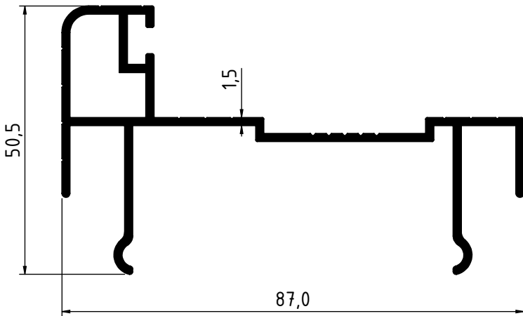
2770 - 0.981 Kg/m
