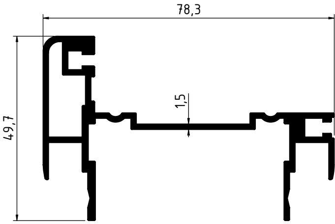
2525 - 1.146 Kg/m
