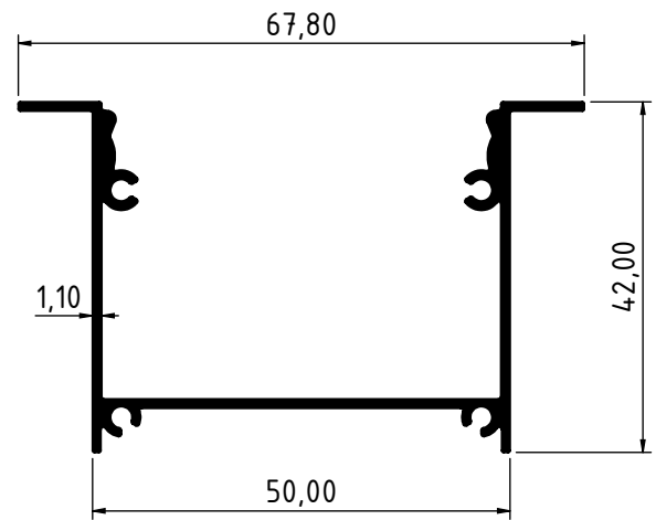
4269 - 0.597 Kg/m
