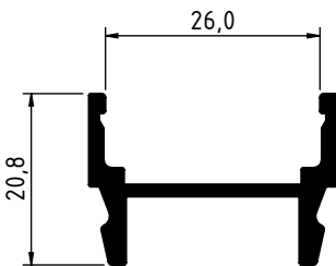
3666 - 0.355 Kg/m
