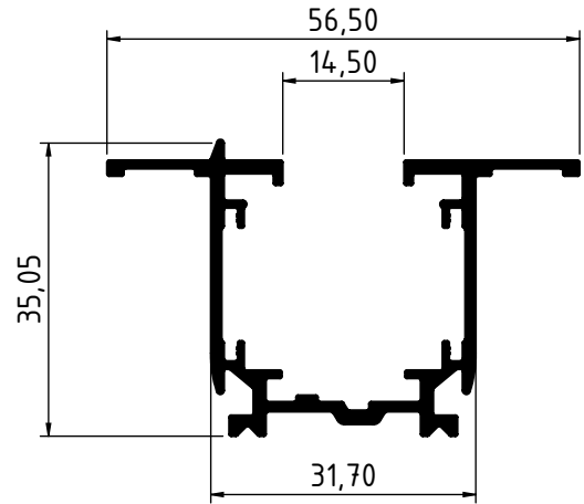
4370 - 0.621 Kg/m
