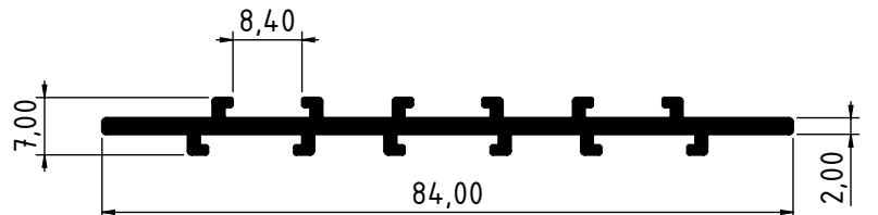
2282 - 0.616 Kg/m
