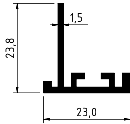
1930 - 0.225 Kg/m
