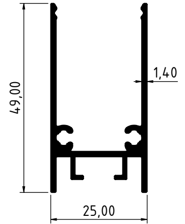
3872 - 0.585 Kg/m
