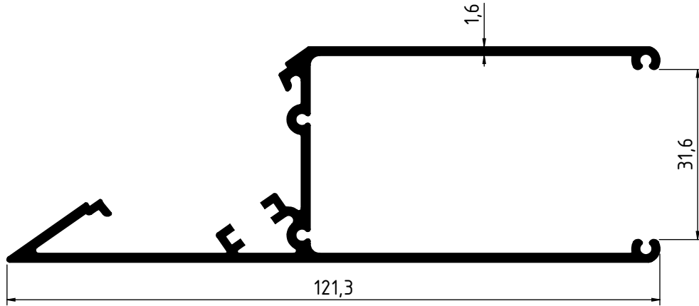
2229 - 0.743 Kg/m
