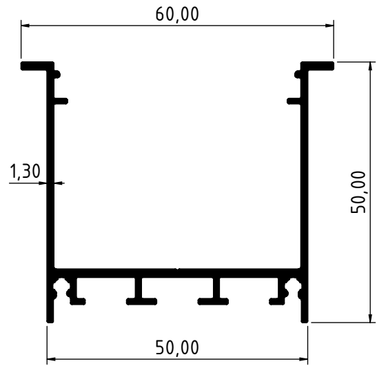
4053 - 0.731 Kg/m
