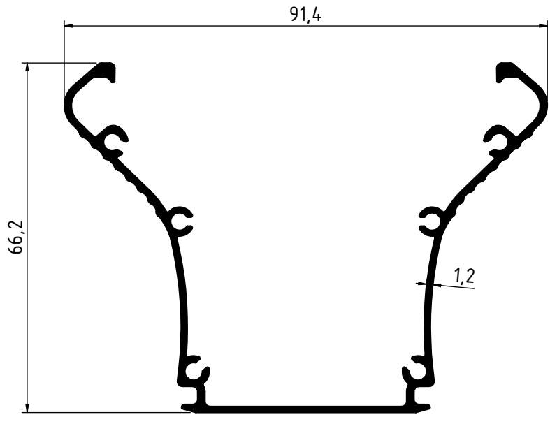
3052 - 0.904 Kg/m
