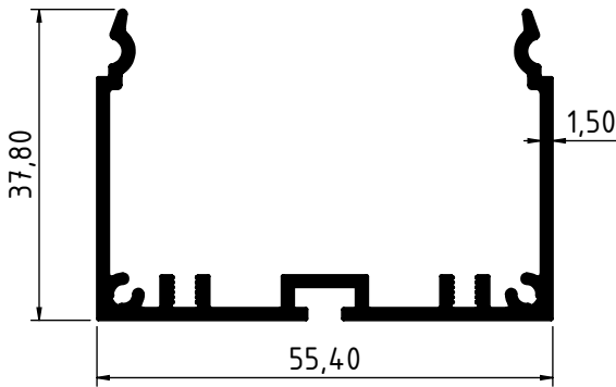
2113 - 0.695 Kg/m
