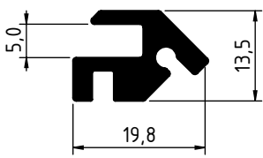
4314 - 0.350 Kg/m
