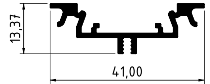
4157 - 0.296 Kg/m
