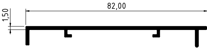
4287 - 0.428 Kg/m
