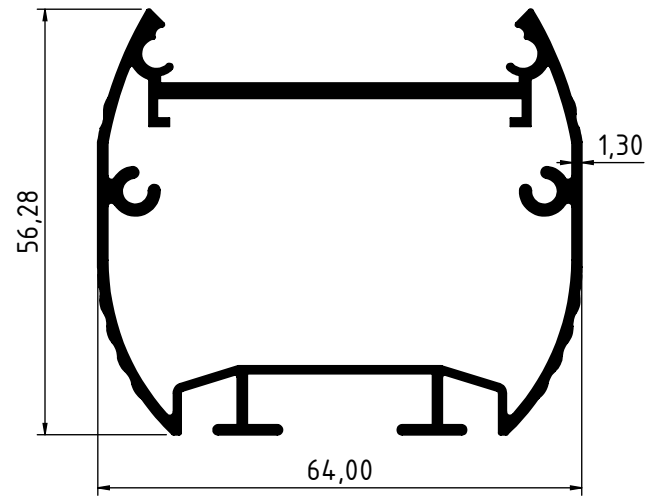
2267 - 1.180 Kg/m
