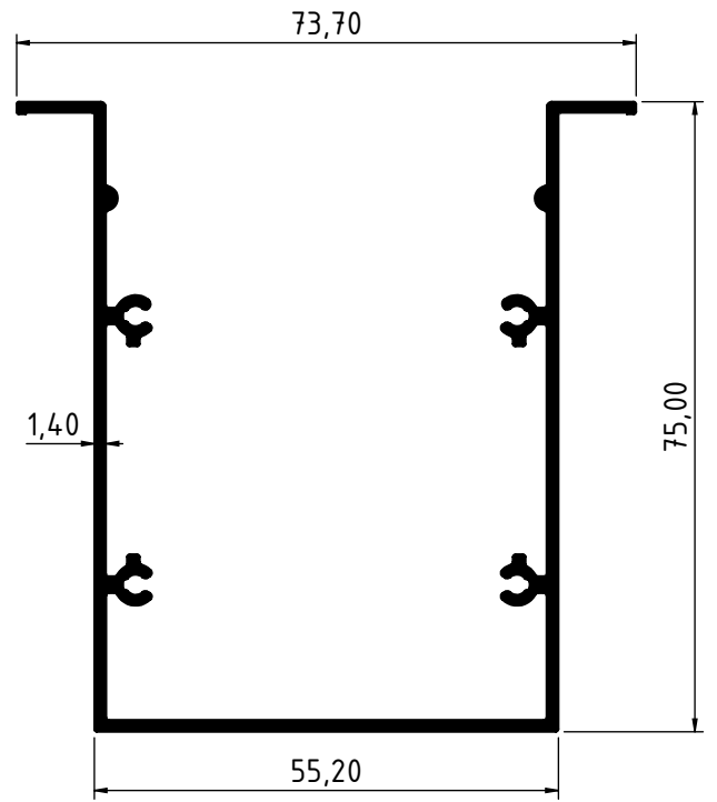
3681 - 1.021 Kg/m
