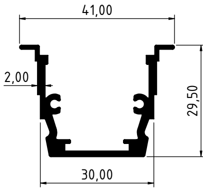
3019 - 0.551 Kg/m
