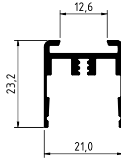
4423 - 0.274 Kg/m
