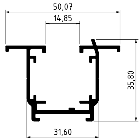
3941 - 0.593 Kg/m
