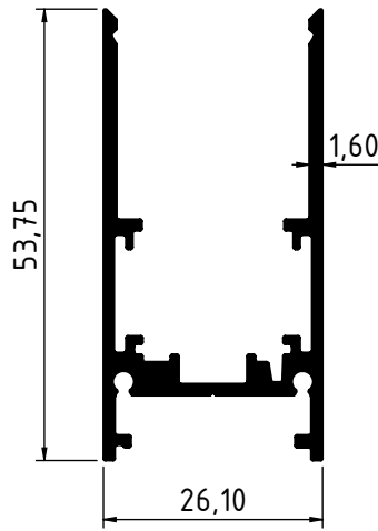
4313 - 0.666 Kg/m
