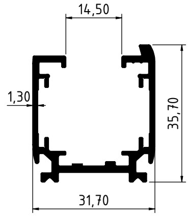
3995 - 0.589 Kg/m
