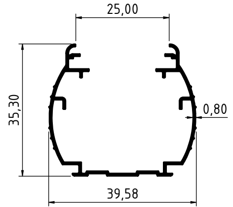
4129 - 0.322 Kg/m
