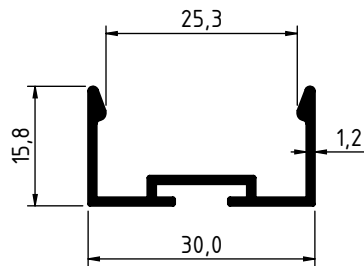
3125 - 0.233 Kg/m
