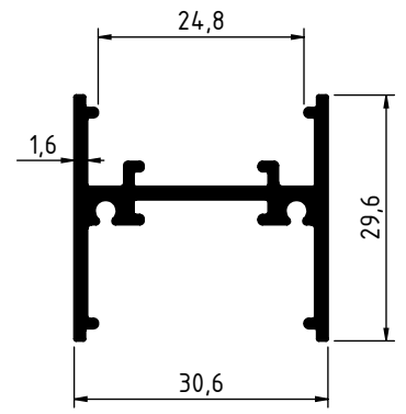
4351 - 0.479 Kg/m
