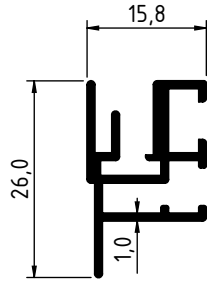
2406 - 0.269 Kg/m
