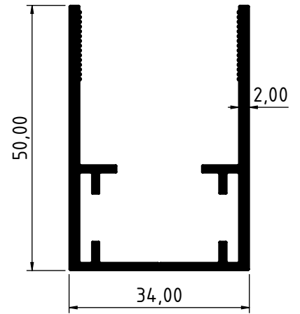
4244 - 0.796 Kg/m
