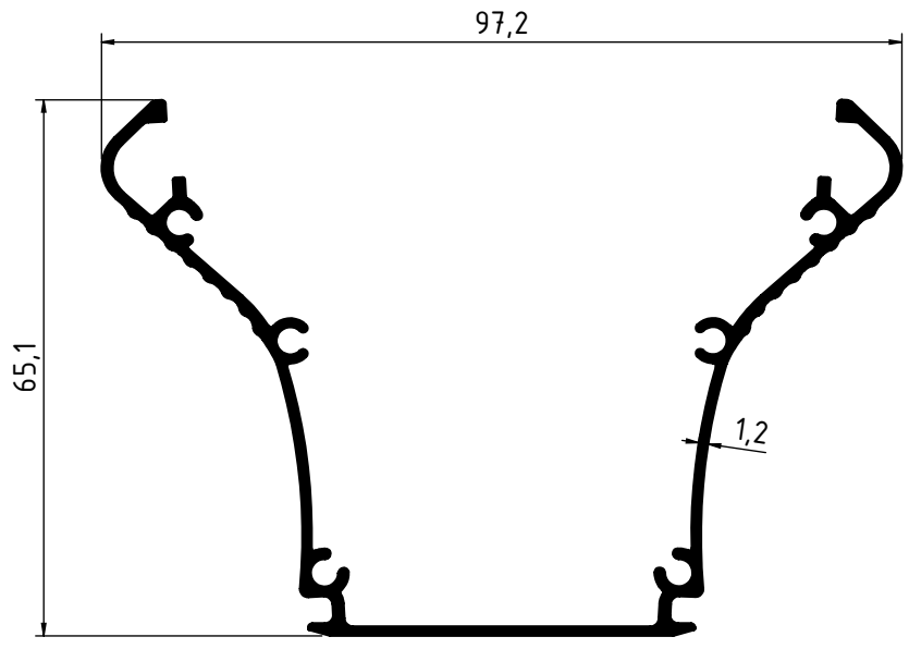
3286 - 0.889 Kg/m
