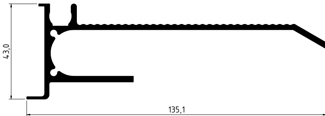
4315 - 1.474 Kg/m
