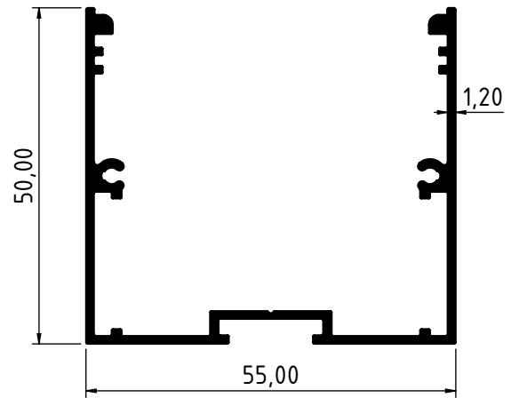
3262 - 0.683 Kg/m
