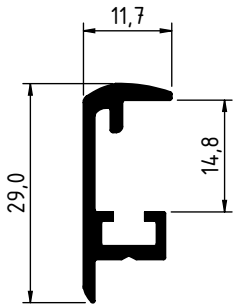
2558 - 0.263 Kg/m
