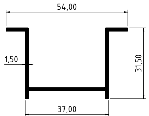
4098 - 0.463 Kg/m
