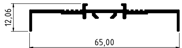
3507 - 0.287 Kg/m
