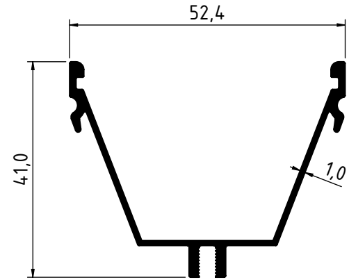
3083 - 0.442 Kg/m
