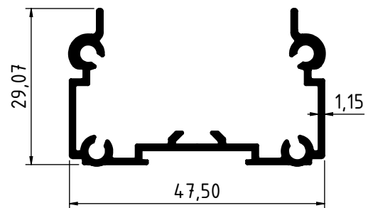
3144 - 0.532 Kg/m
