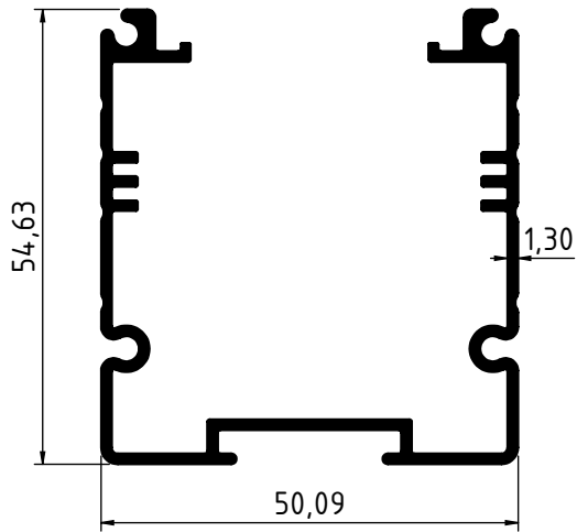
3818 - 0.845 Kg/m
