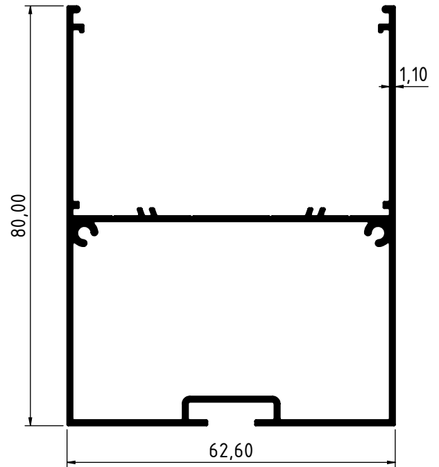
4304 - 0.993 Kg/m
