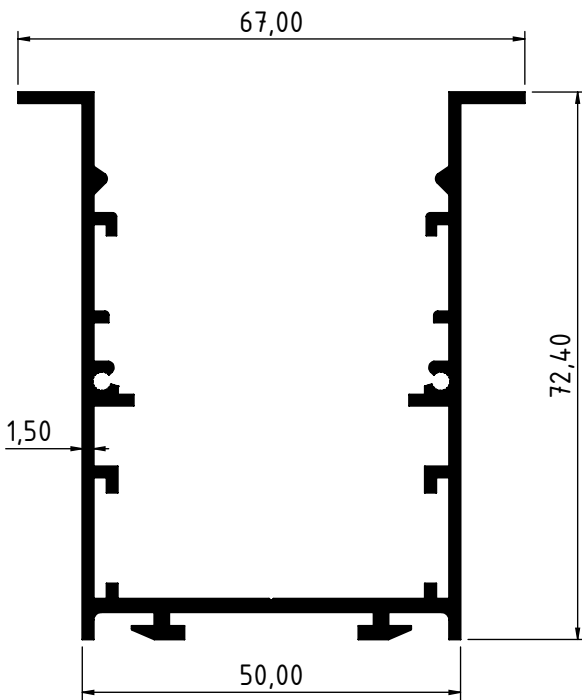
2609 - 1.158 Kg/m
