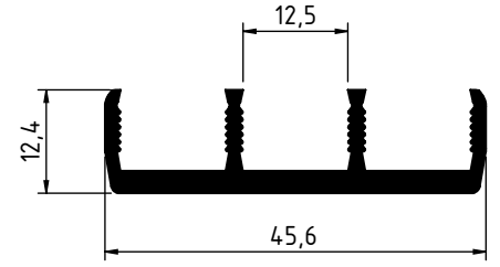
2762 - 0.491 Kg/m
