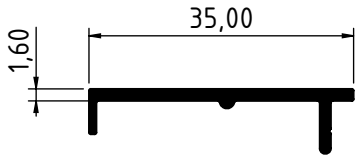
4084 - 0.195 Kg/m
