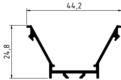
3133 - 0.285 Kg/m
