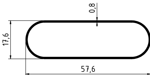
3298 - 0.287 Kg/m
