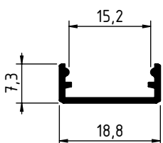
3822 - 0.095 Kg/m
