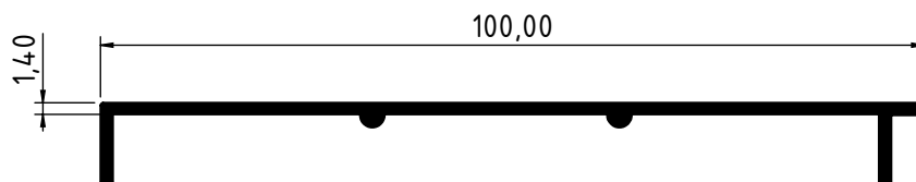
2613 - 0.471 Kg/m
