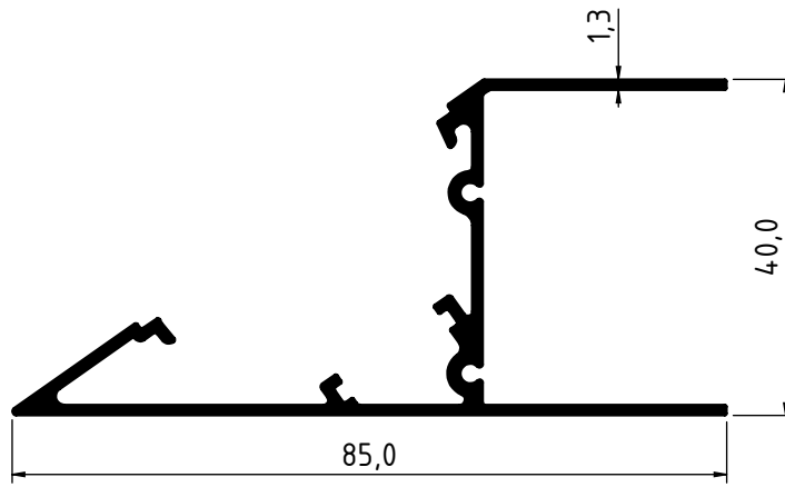
2229 - 0.743 Kg/m
