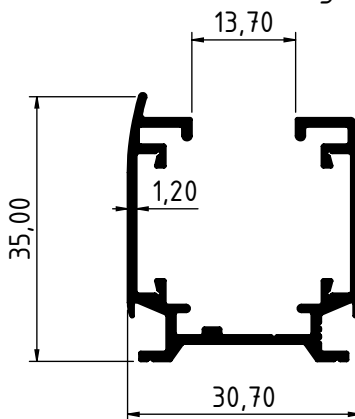
4347 - 0.473 Kg/m
