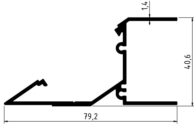
3239 - 0.735 Kg/m
