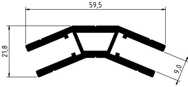
2181 - 0.934 Kg/m
