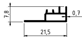
3292 - 0.090 Kg/m
