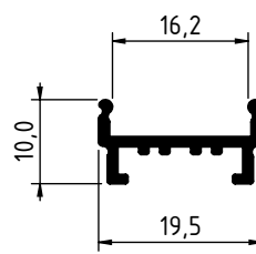
2837 - 0.141 Kg/m
