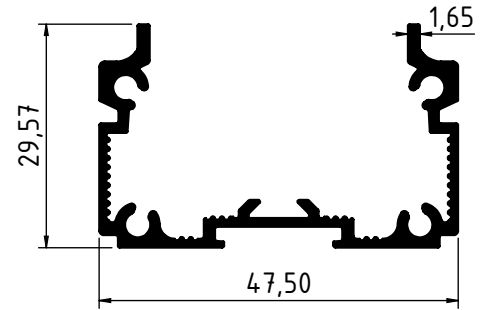
4028 - 0.581 Kg/m
