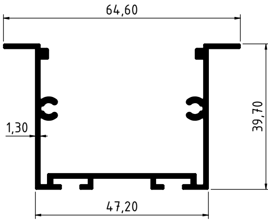
2715 - 0.702 Kg/m
