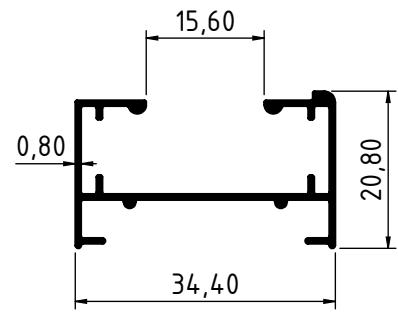
4424 - 0.252 Kg/m
