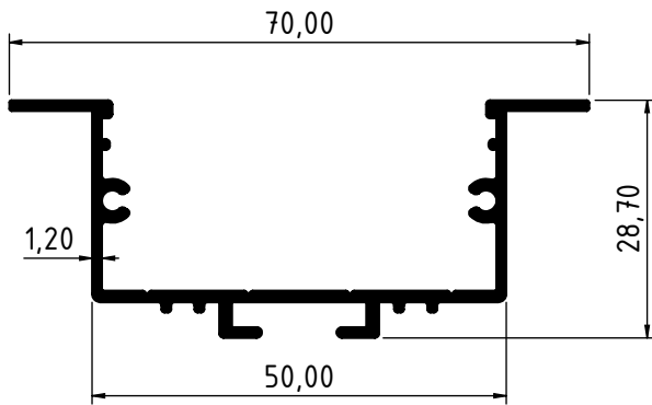
3154 - 0.561 Kg/m
