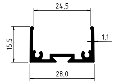
2741 - 0.260 Kg/m
