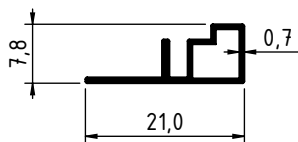
3132 - 0.095 Kg/m
