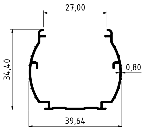
4128 - 0.265 Kg/m
