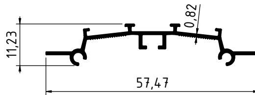
3300 - 0.217 Kg/m
