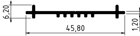
3720 - 0.210 Kg/m
