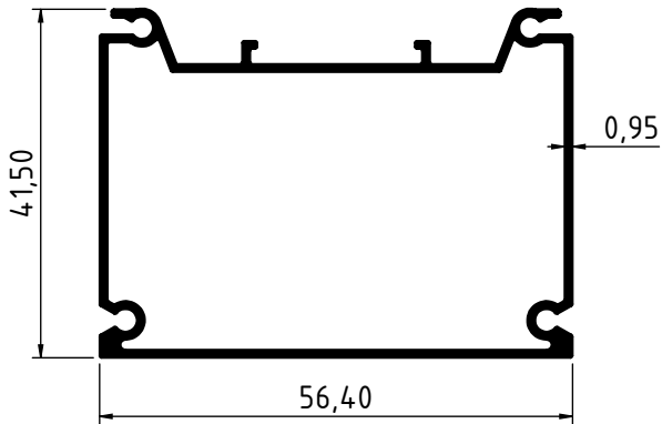
4114 - 0.605 Kg/m
