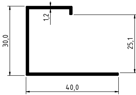
3201 - 0.293 Kg/m
