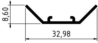
4197 - 0.122 Kg/m
