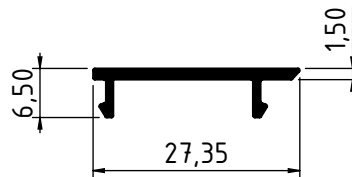
3651 - 0.144 Kg/m
