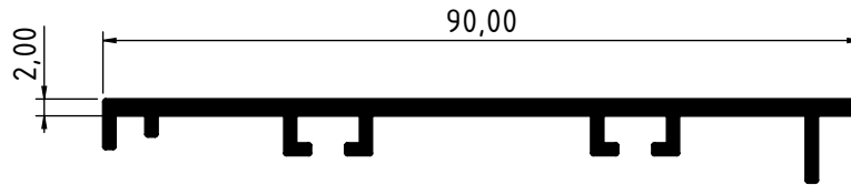
2716 - 0.653 Kg/m
