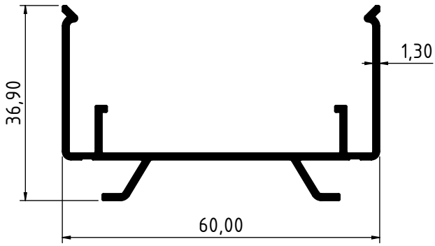
3497 - 0.569 Kg/m
