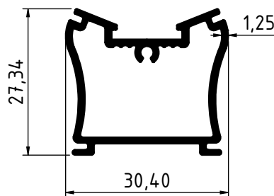
2530 - 0.436 Kg/m
