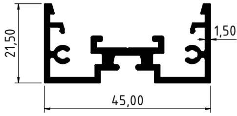
1284 - 0.648 Kg/m
