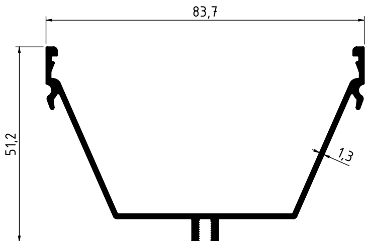
3383 - 0.633 Kg/m
