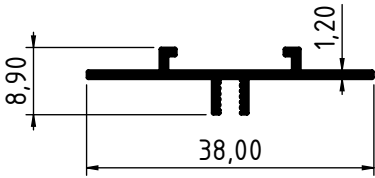
3195 - 0.178 Kg/m
