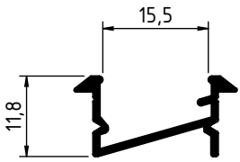
3179 - 0.144 Kg/m
