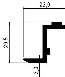
3649 - 0.240 Kg/m
