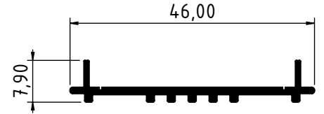
2523 - 0.239 Kg/m
