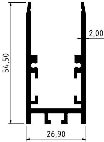
3135 - 0.892 Kg/m
