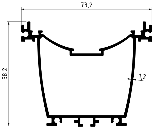
2559 - 1.067 Kg/m
