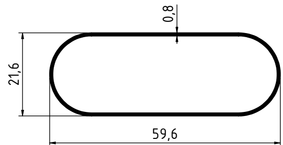
3311 - 0.306 Kg/m
