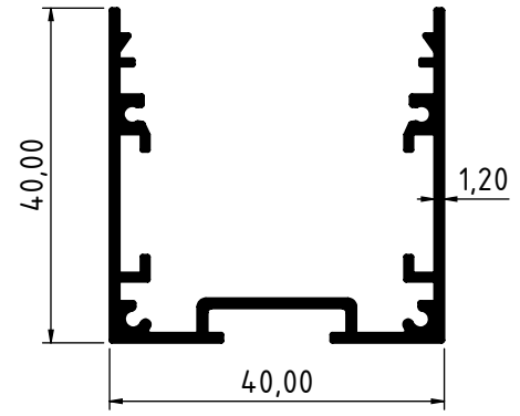
2818 - 0.580 Kg/m
