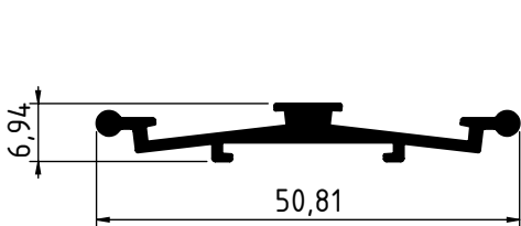
3065 - 0.312 Kg/m
