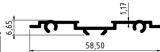
3317 - 0.298 Kg/m
