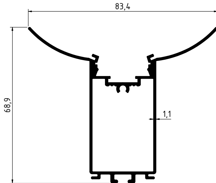
2617 - 0.870 Kg/m
