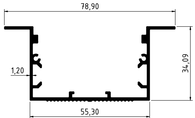
2541 - 0.688 Kg/m
