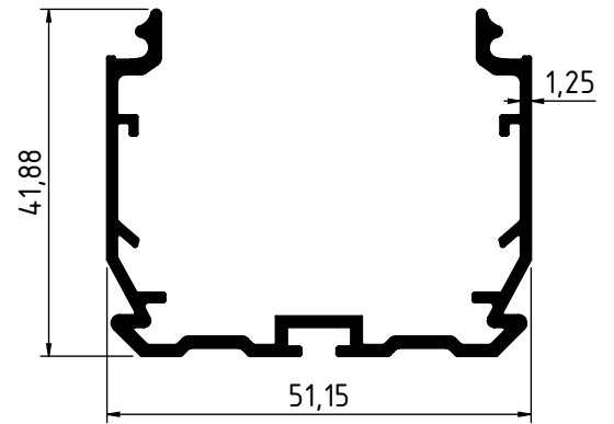
2697 - 0.659 Kg/m
