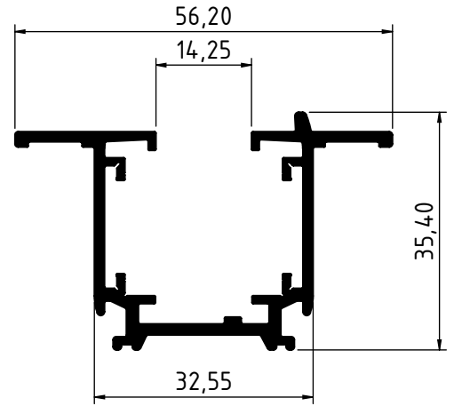
4142 - 0.707 Kg/m
