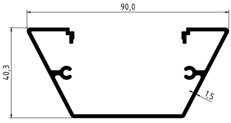
4159 - 0.900 Kg/m
