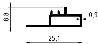
3744 - 0.123 Kg/m
