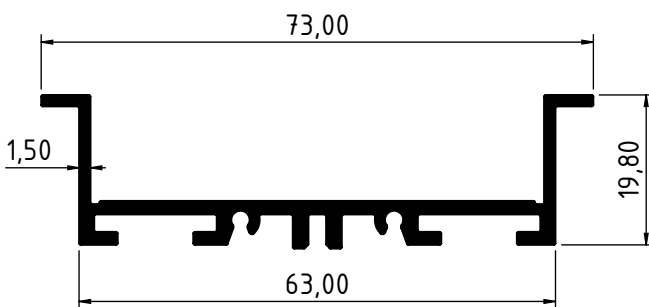
4319 - 0,636 Kg/m
