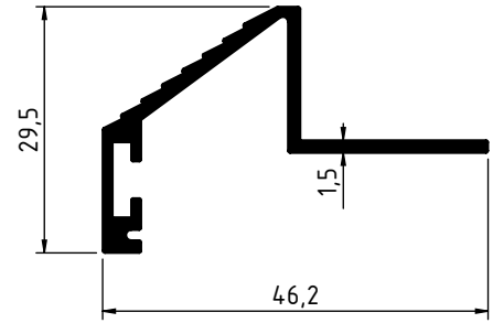
3069 - 0.393 Kg/m
