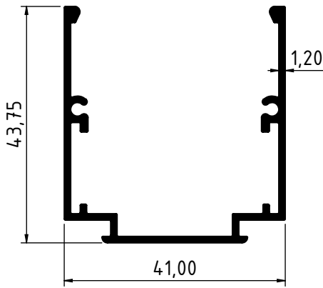
4156 - 0.514 Kg/m
