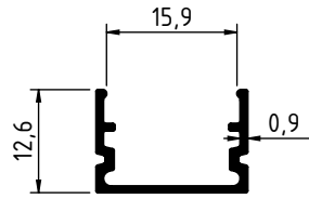
4124 - 0.120 Kg/m
