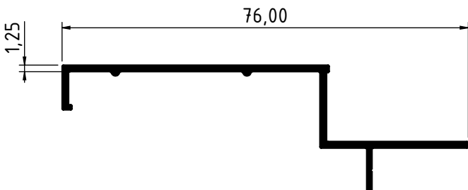
4218 - 0.361 Kg/m
