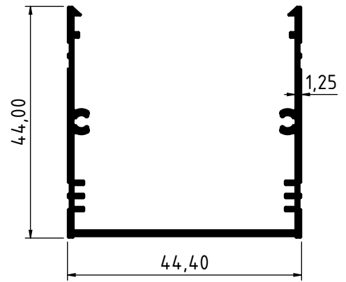
2798 - 0.515 Kg/m
