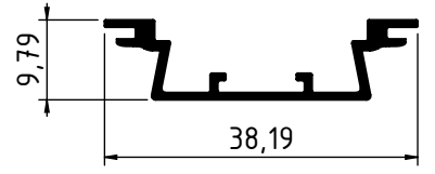
4133 - 0.196 Kg/m
