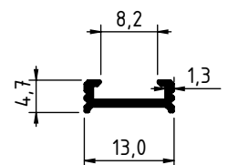
2343 - 0.064 Kg/m
