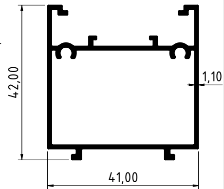
2668 - 0.596 Kg/m
