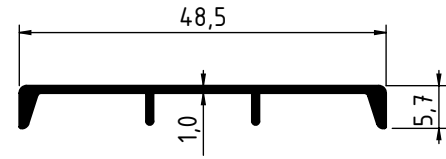
2422 - 0.196 Kg/m
