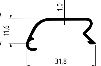
4093 - 0.162 Kg/m
