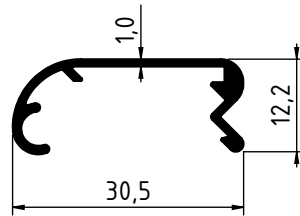
2234 - 0.189 Kg/m
