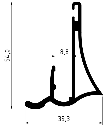
2737 - 0.690 Kg/m
