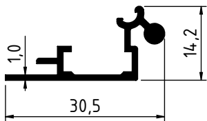
2233 - 0.194 Kg/m
