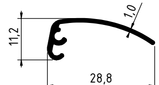
2644 - 0.132Kg/m
