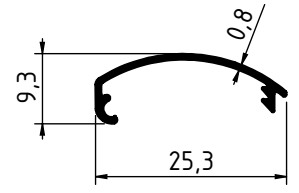
3357 - 0.088 Kg/m
