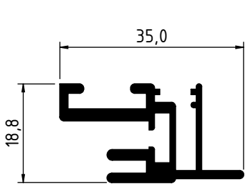
2090 - 0.475 Kg/m
