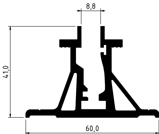
1980 - 1.415 Kg/m
