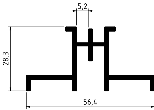
3029 - 0.700 Kg/m
