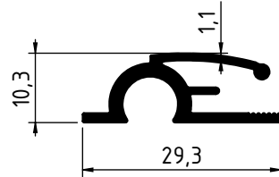
1942 - 0.257 Kg/m
