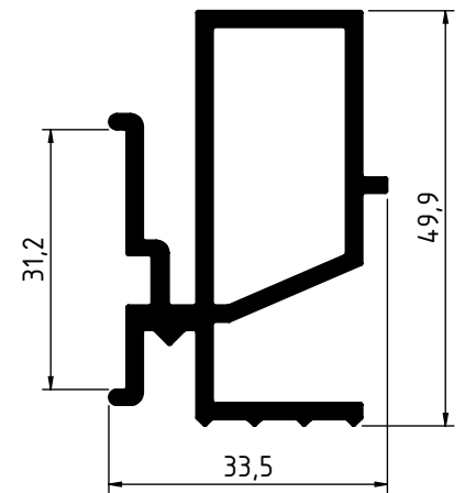
4225 - 1.160 Kg/m
