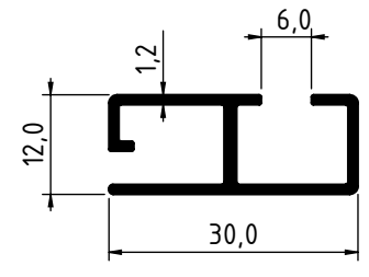
4121 - 0.268 Kg/m
