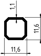
2313 - 0.114 Kg/m
