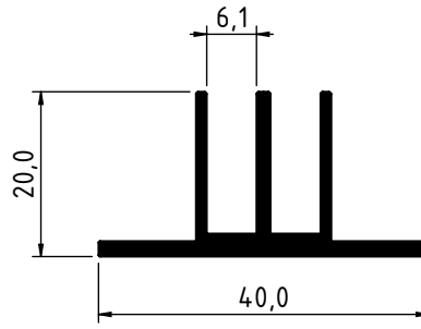
1006 - 0.446 Kg/m
