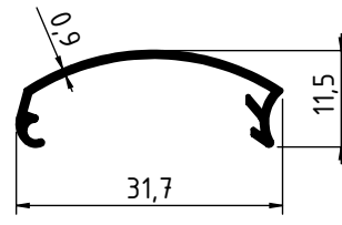
2350 - 0.129 Kg/m
