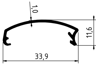
2080 - 0.189 Kg/m
