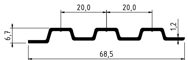
2084 - 0.288 Kg/m
