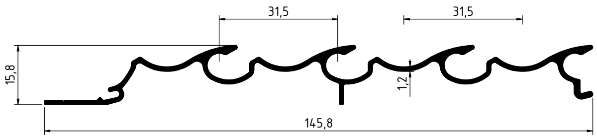
4118 - 0.790 Kg/m
