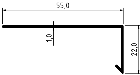
1952 - 0.217 Kg/m
