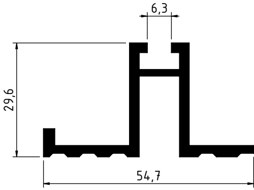
2491 - 0.773 Kg/m
