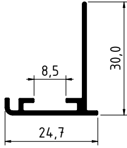
4554 - 0,207 Kg/m
