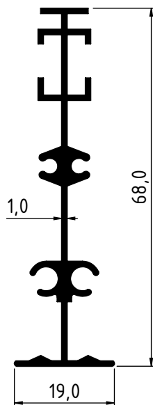
2312 - 0.524 Kg/m
