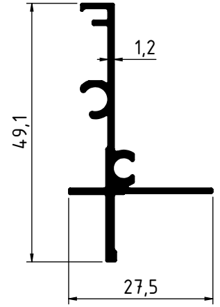
4298 - 0.352 Kg/m
