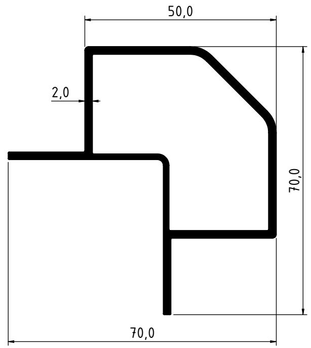
2265 - 1.136 Kg/m
