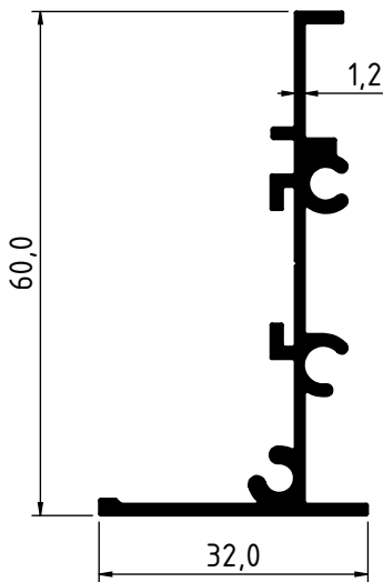
1850 - 0.542 Kg/m
