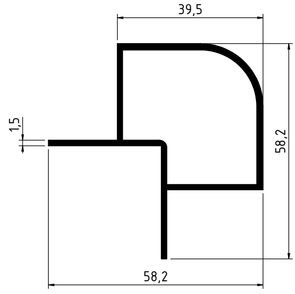
2249 - 0.765 Kg/m
