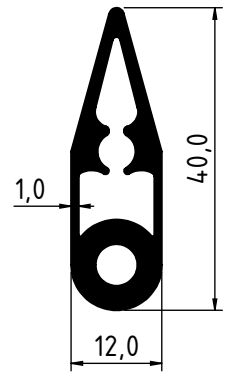
2404 - 0.561 Kg/m
