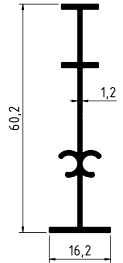
1849 - 0.380 Kg/m
