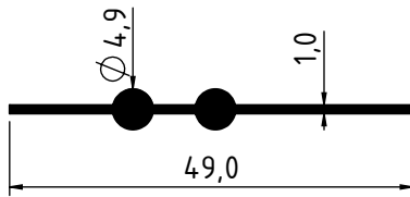
1210 - 0.209 Kg/m
