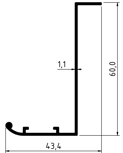
1945 - 0.347 Kg/m
