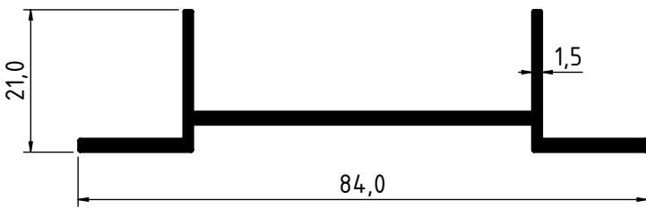
2402 - 0.610 Kg/m
