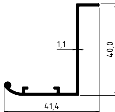
1817 - 0.282 Kg/m
