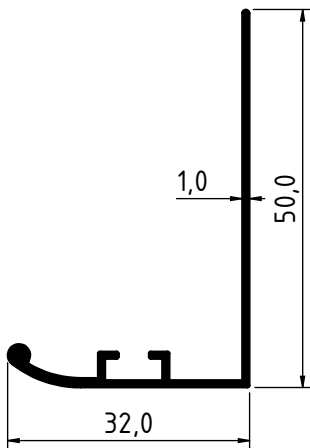
2508 - 0.274 Kg/m
