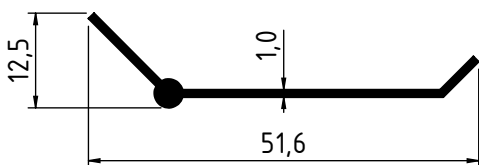
2219 - 0.177 Kg/m
