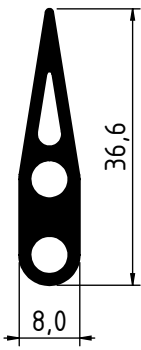
2391 - 0.396 Kg/m
