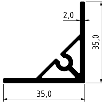
2490 - 0.545 Kg/m
