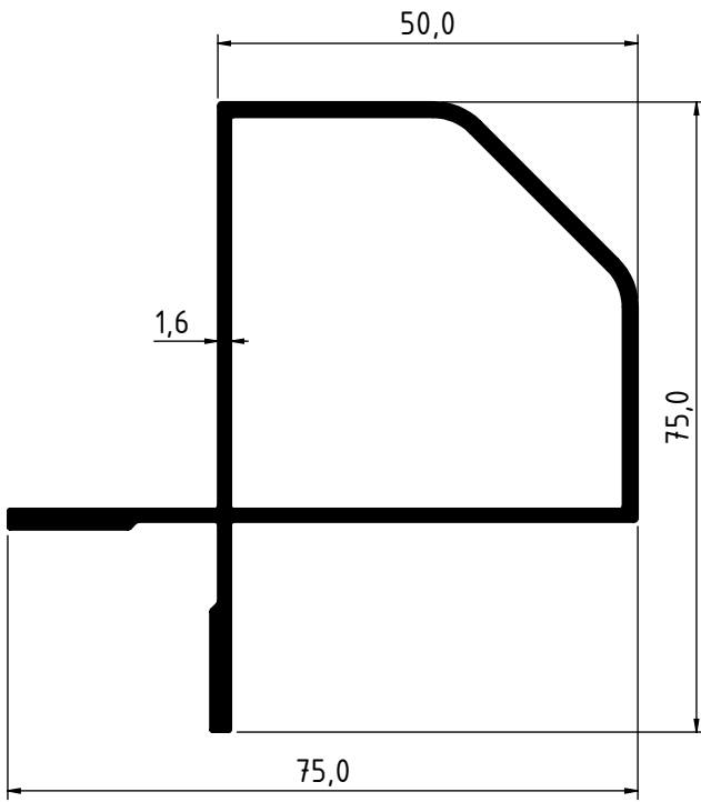
3494 - 1.119 Kg/m
