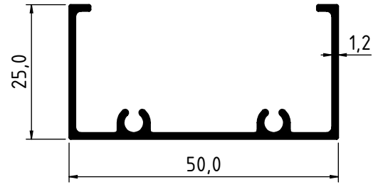
2213 - 0.407 Kg/m
