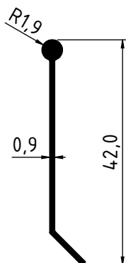
4552 - 0.129 Kg/m
