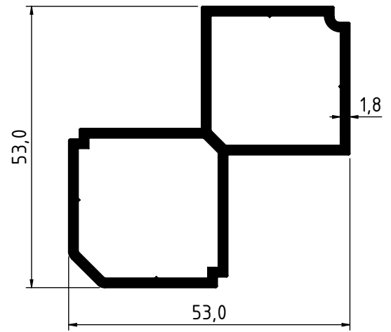
1947 - 0.998 Kg/m
