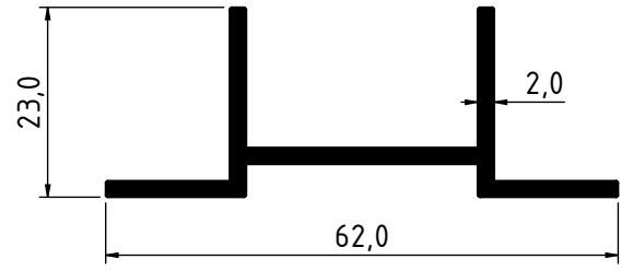
2401 - 0.564 Kg/m
