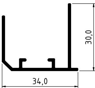
1845 - 0.315 Kg/m
