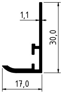
2542 - 0.185 Kg/m
