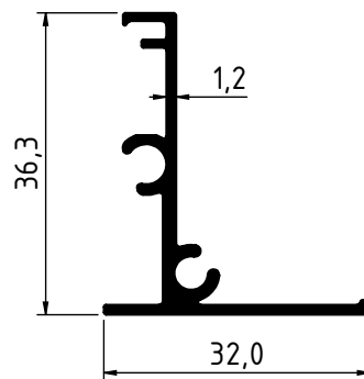
4259 - 0.332 Kg/m
