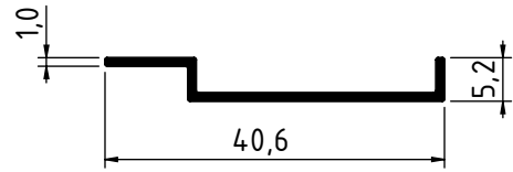
4557 - 0,133 Kg/m
