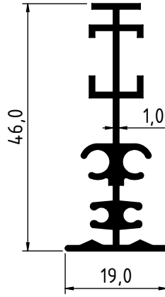
2067 - 0.437 Kg/m
