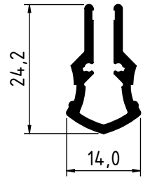
1997 - 0.261 Kg/m
