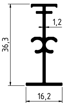
4260 - 0.280 Kg/m
