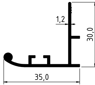
2596 - 0.285 Kg/m
