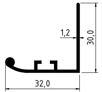
2048 - 0.326 Kg/m
