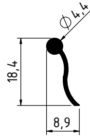
2068 - 0.087 Kg/m
