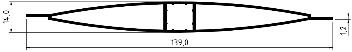
2071 - 0.805 Kg/m
