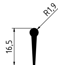
4550 - 0.065 Kg/m
