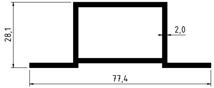
2250 - 0.900 Kg/m
