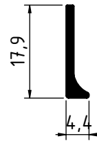
1876 - 0.090 Kg/m
