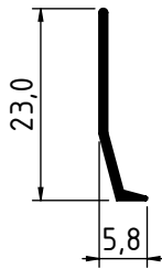
2046 - 0.071 Kg/m
