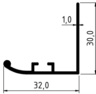
2507 - 0.220 Kg/m
