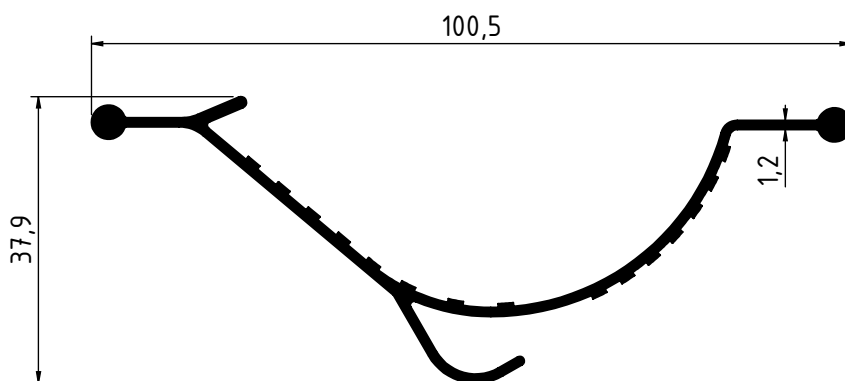
2227 - 0.597 Kg/m
