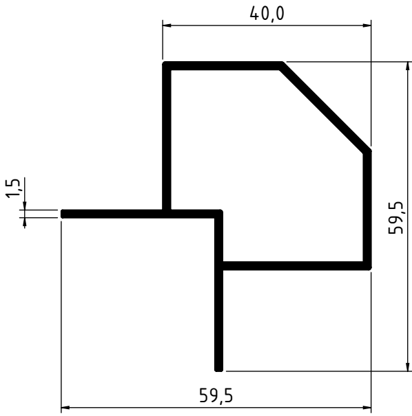
2549 - 0.746 Kg/m
