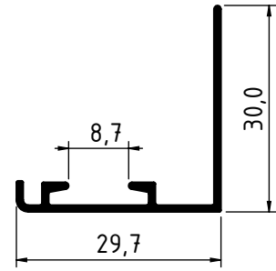
4555 - 0,203 Kg/m
