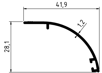
1997 - 0.261 Kg/m
