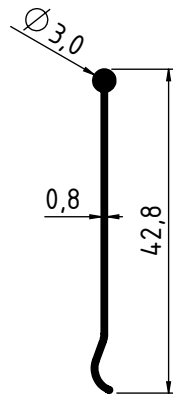
1984 - 0.109 Kg/m
