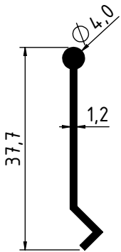
1946 - 0.155 Kg/m
