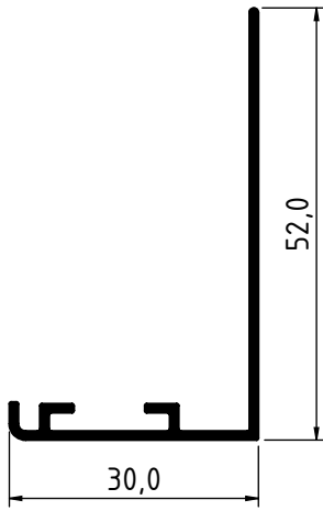
4556 - 0,287 Kg/m
