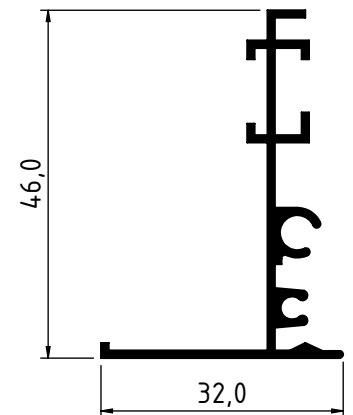
2066 - 0.366 Kg/m
