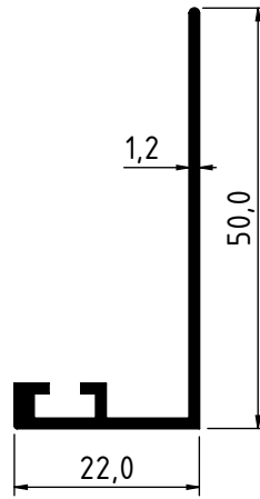
2047 - 0.280 Kg/m
