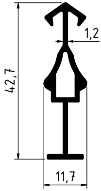
2179 - 0.331 Kg/m
