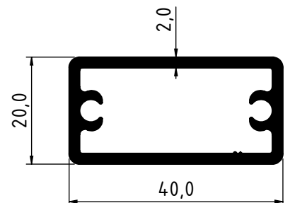
1859 - 0.686 Kg/m
