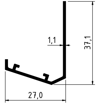
1939 - 0.220 Kg/m
