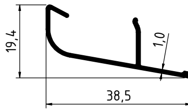
1827 - 0.190 Kg/m
