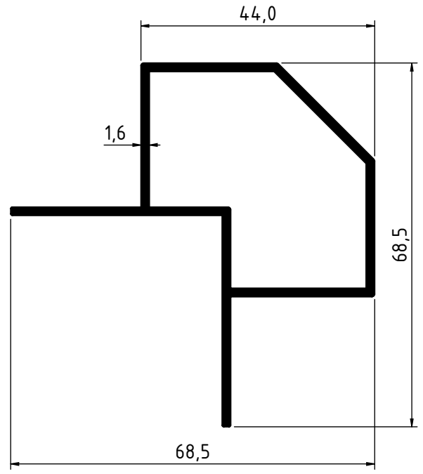
2362 - 0.903 Kg/m
