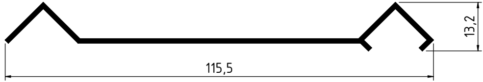
2196 - 0.448 Kg/m
