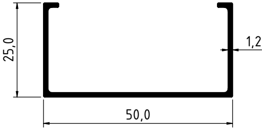
2214 - 0.339 Kg/m
