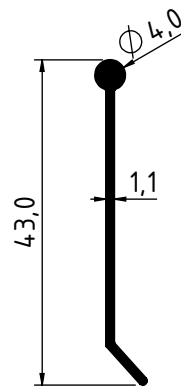
2548 - 0.158 Kg/m
