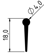
2225 - 0.087 Kg/m
