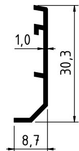
2211 - 0.122 Kg/m
