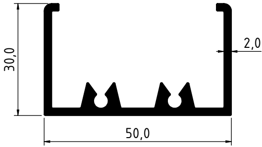
1267 - 0.789 Kg/m
