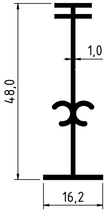
1815 - 0.293 Kg/m
