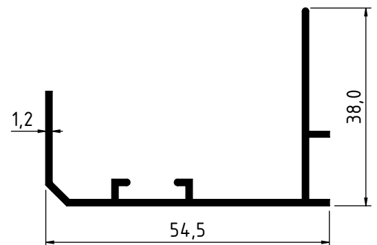
2315 - 0.410 Kg/m
