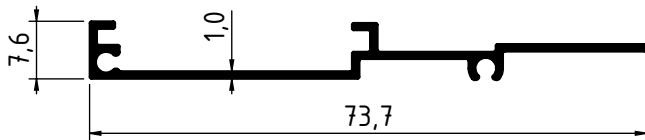
2477 - 0.280 Kg/m
