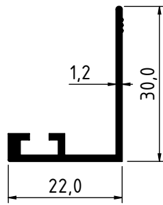
2118 - 0.217 Kg/m
