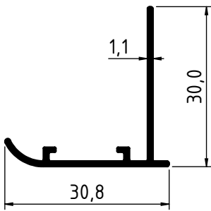
1812 - 0.206 Kg/m
