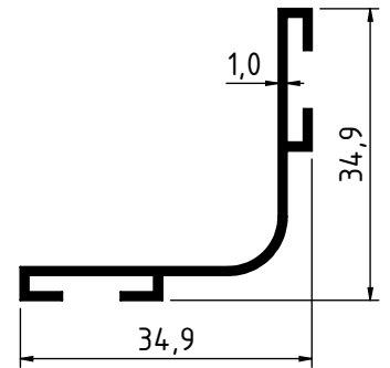
2212 - 0.242 Kg/m
