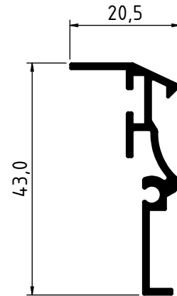
2366 - 0.320 Kg/m
