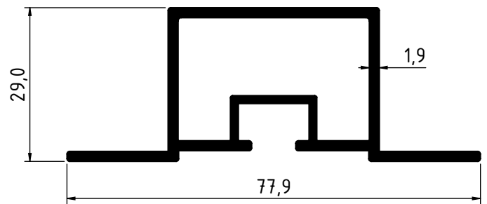
2811 - 0.946 Kg/m
