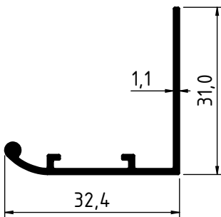
1813 - 0.225 Kg/m
