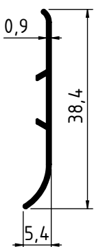
2374 - 0.112 Kg/m
