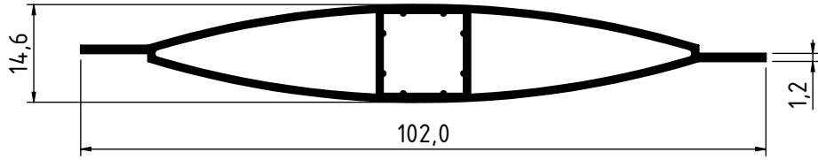
2051 - 0.610 Kg/m
