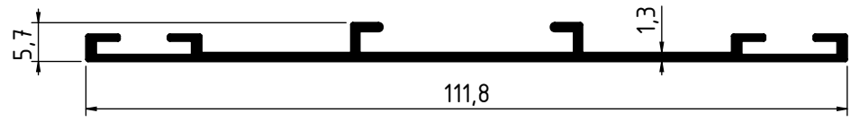
2377 - 0.507 Kg/m
