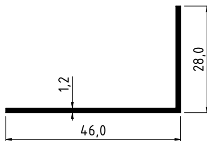
2070 - 0.239 Kg/m
