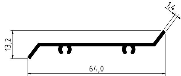
1209 - 0.326 Kg/m
