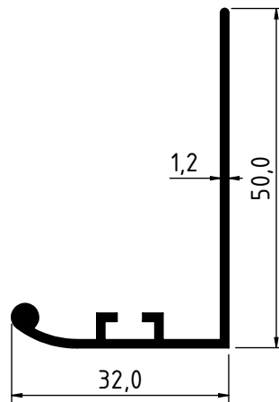
2049 - 0.326 Kg/m
