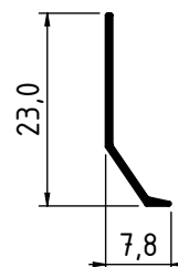
4551 - 0.057 Kg/m
