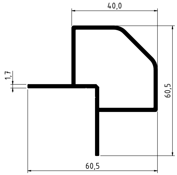
2812 - 0.845 Kg/m
