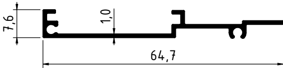
1211 - 0.255 Kg/m
