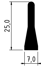
1876 - 0.090 Kg/m
