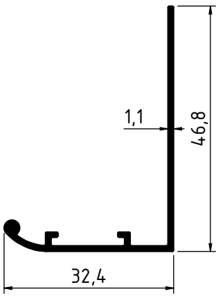
1846 - 0.273 Kg/m
