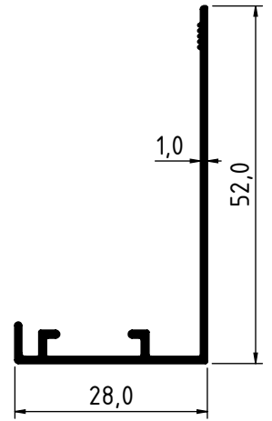
4356 - 0.263 Kg/m
