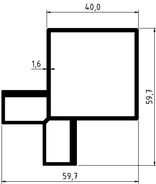
1231 - 1.187 Kg/m
