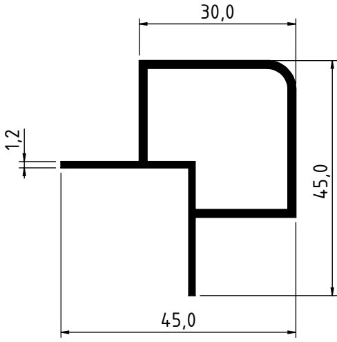
2248 - 0.540 Kg/m
