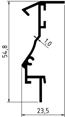
1916 - 0.366 Kg/m
