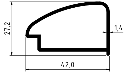
2930 - 0.483 Kg/m
