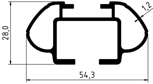
4303 - 0.698 Kg/m
