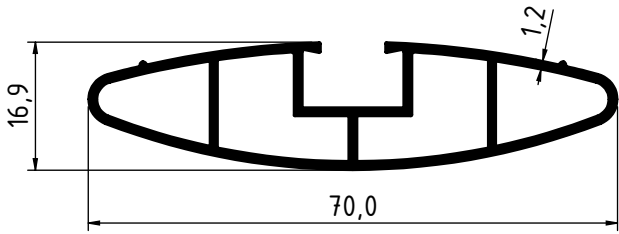
2157 - 0.636 Kg/m
