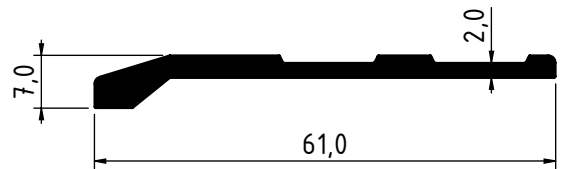
2576 - 0.467 Kg/m
