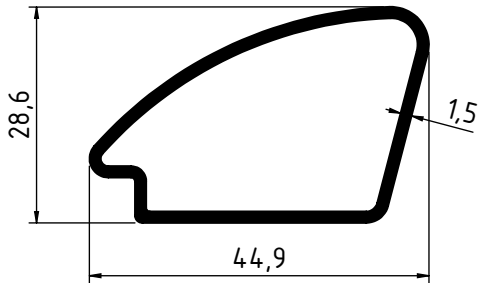
2028 - 0.487 Kg/m
