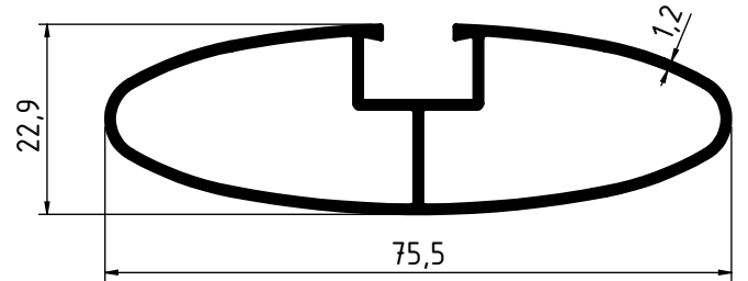
2166 - 0.649 Kg/m
