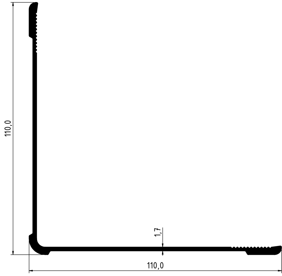
4452 - 1.142 Kg/m
