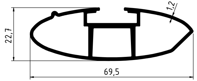
3889 - 0.755 Kg/m
