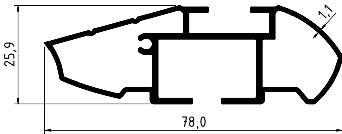
3975 - 0.848 Kg/m
