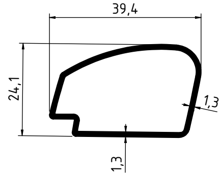
4155 - 0.376 Kg/m
