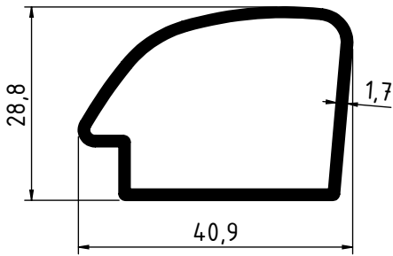
2027 - 0.505 Kg/m
