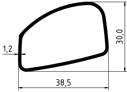
2195 - 0.358 Kg/m
