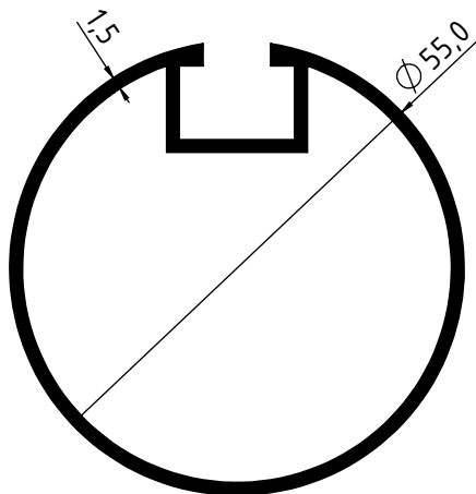
2013 - 0.807 Kg/m
