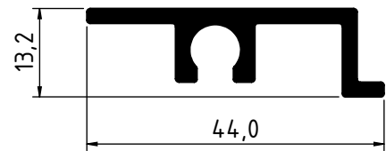
2874 - 0.467 Kg/m
